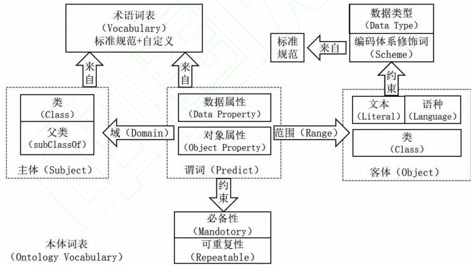
图 2 本体应用纲要中术语词表的组成和定义
