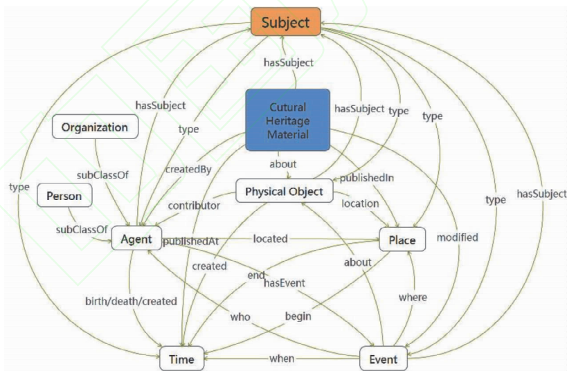
图3 一体化本体的知识融通模型
