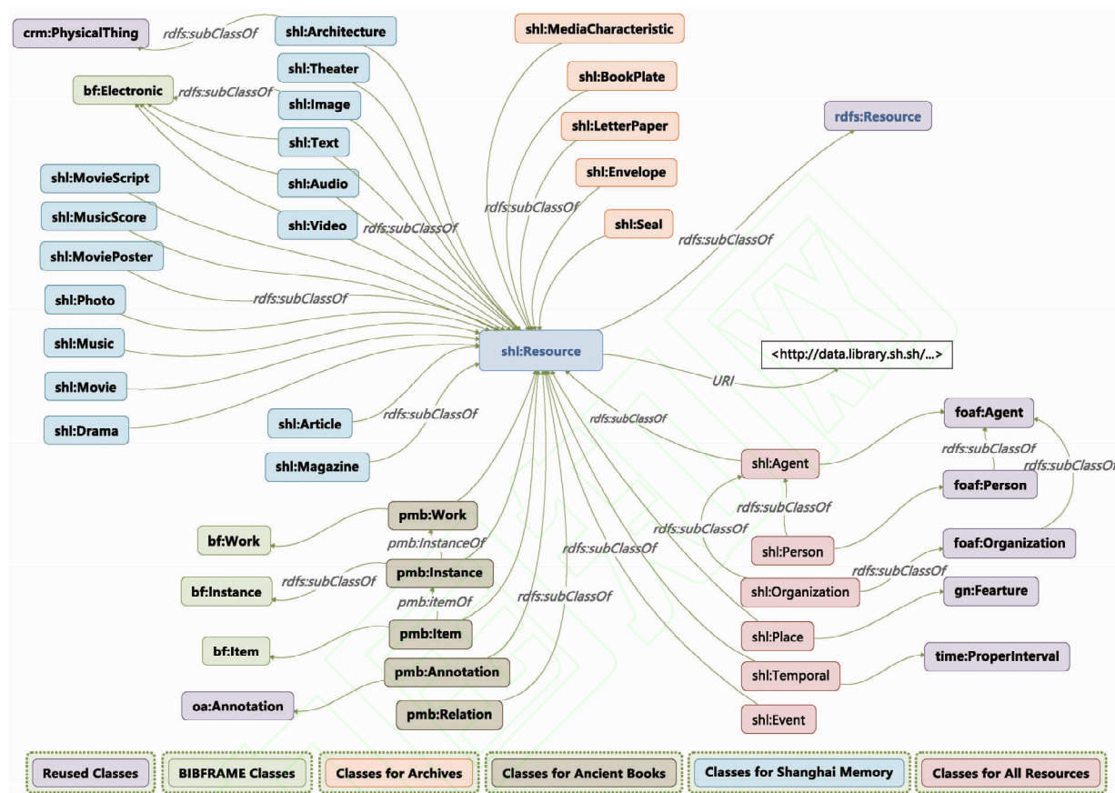
图4 一体化本体中类的复用和继承关系
