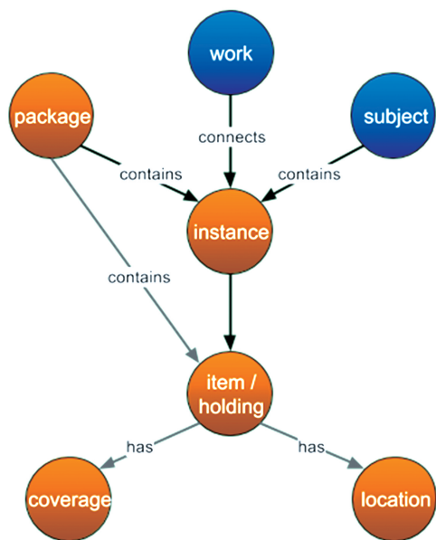
图 4 Codex 的数据模型 ①
