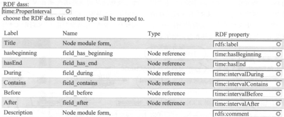
图4 定义内容模型和 RDF 数据模型之间的映射
