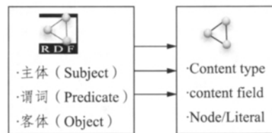
图 1 RDF 数据模型与 Drupal 内容模型的映射关系
