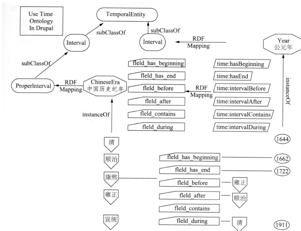
图3 定义内容结构和本体映射方案
